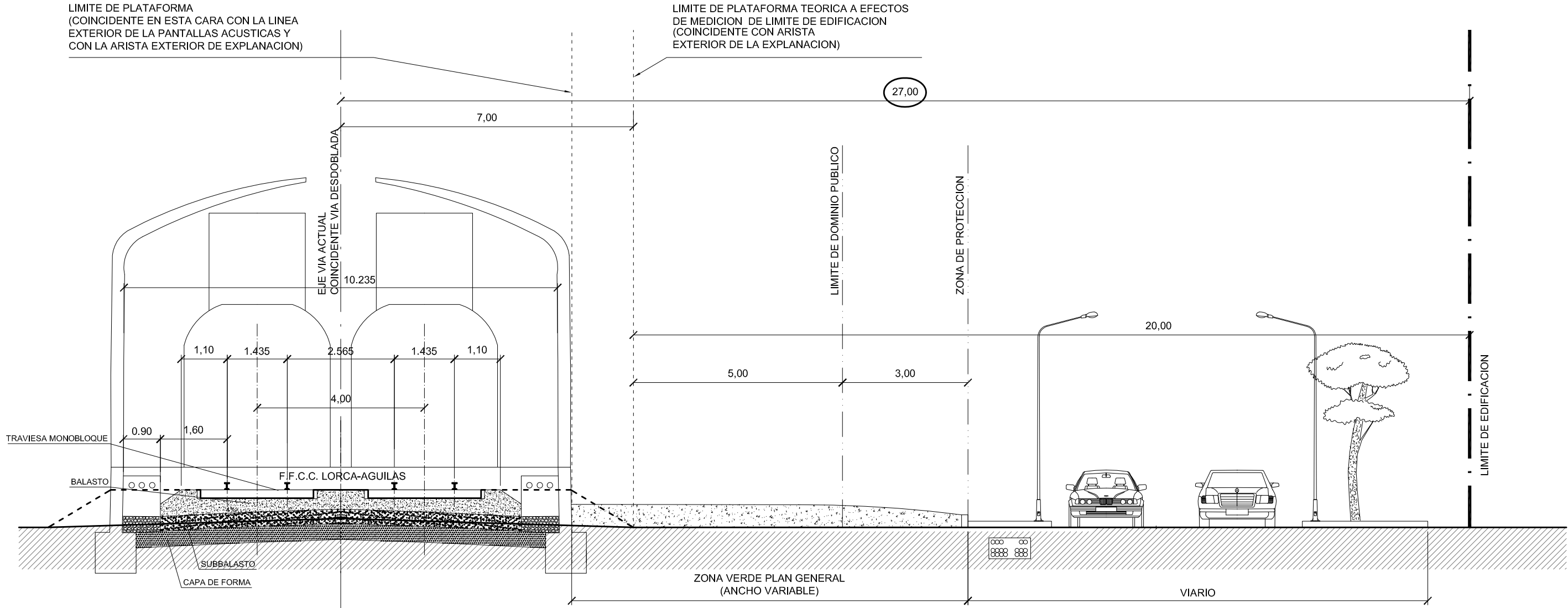
SECCION TRANSVERSAL TEORICA PARA LA DEFINICION DEL LIMITE DE EDIFICACION (27 mts. a eje vía actual). (EN CONFORMIDAD CON OTRO INFORME EMITIDO PARA EL SECTOR "LORCA S-9.R." EXPTE. AA 56/06) (EN CONFORMIDAD CON LOS ARTS. 25, 26, 27 Y 30 DEL R.D. /2004. REGLAMENTO FERROVIARIO Y ORDEN FOM / 2005 DEL 6 DE JULIO)
