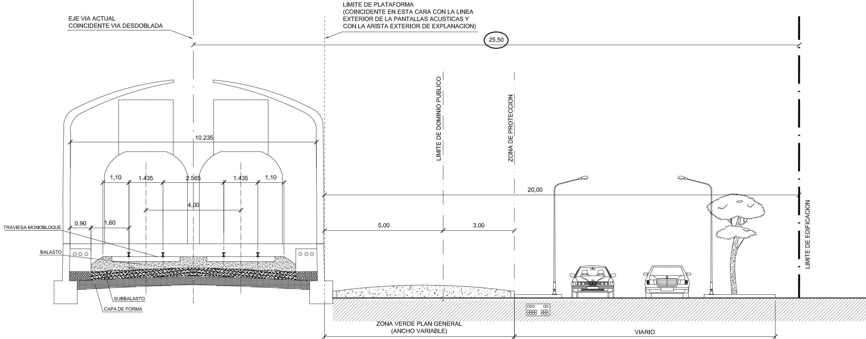
SECCION TRANSVERSAL SEGUN ESTUDIO INFORMATIVO CORREDOR MEDITERRANEO, SEPARATA AYTO. DE LORCA (APROBADO DEFINITIVAMENTE). (ANCHO DE PLATAFORMA = ANCHO PANTALLA ACUSTICA) (LIMITE DE EDIFICACION EN ESTE CASO = 25,5 mts. EJE VIA ACTUAL)
